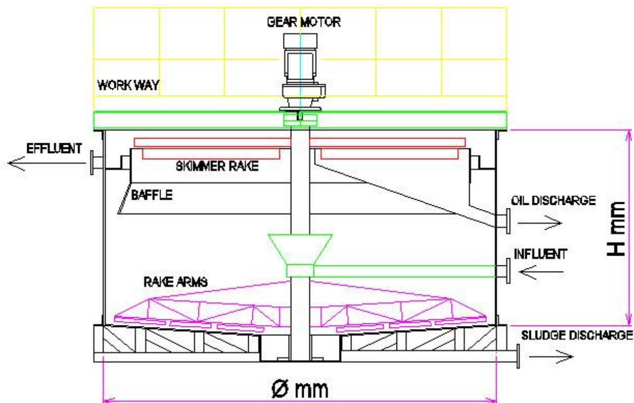
Kết Cấu Bể Tuyển Nổi Hình Tròn
