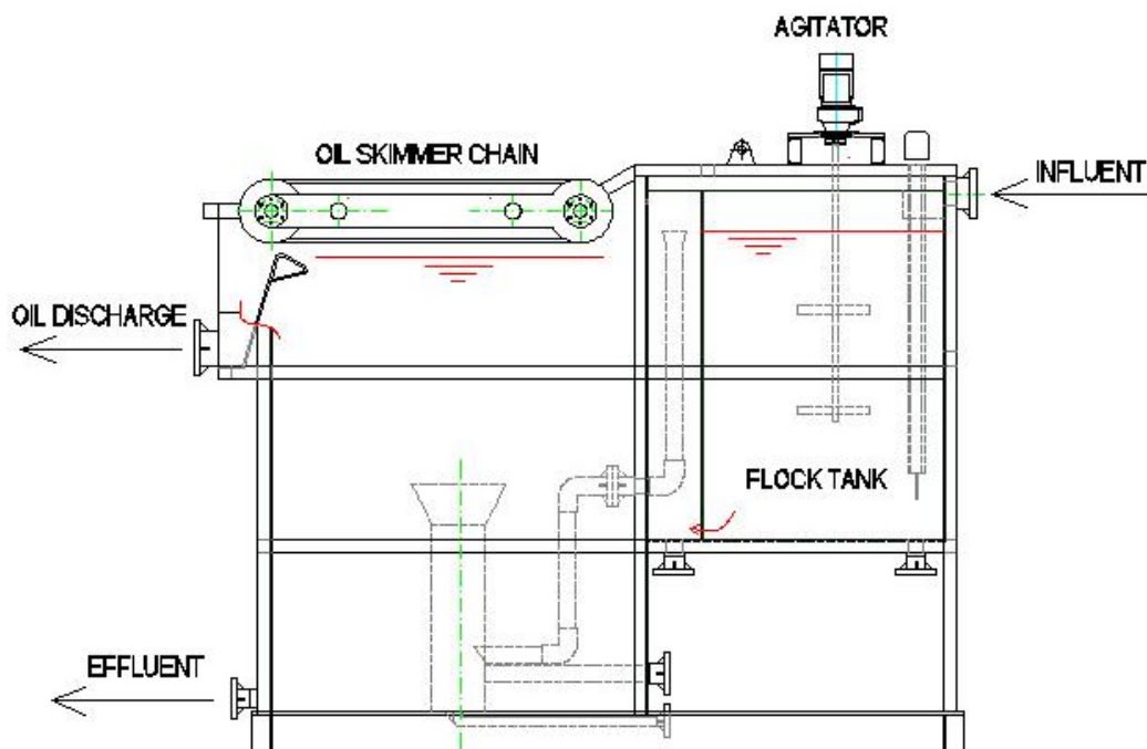
Bể Tuyển Nổi Hình Hộp
