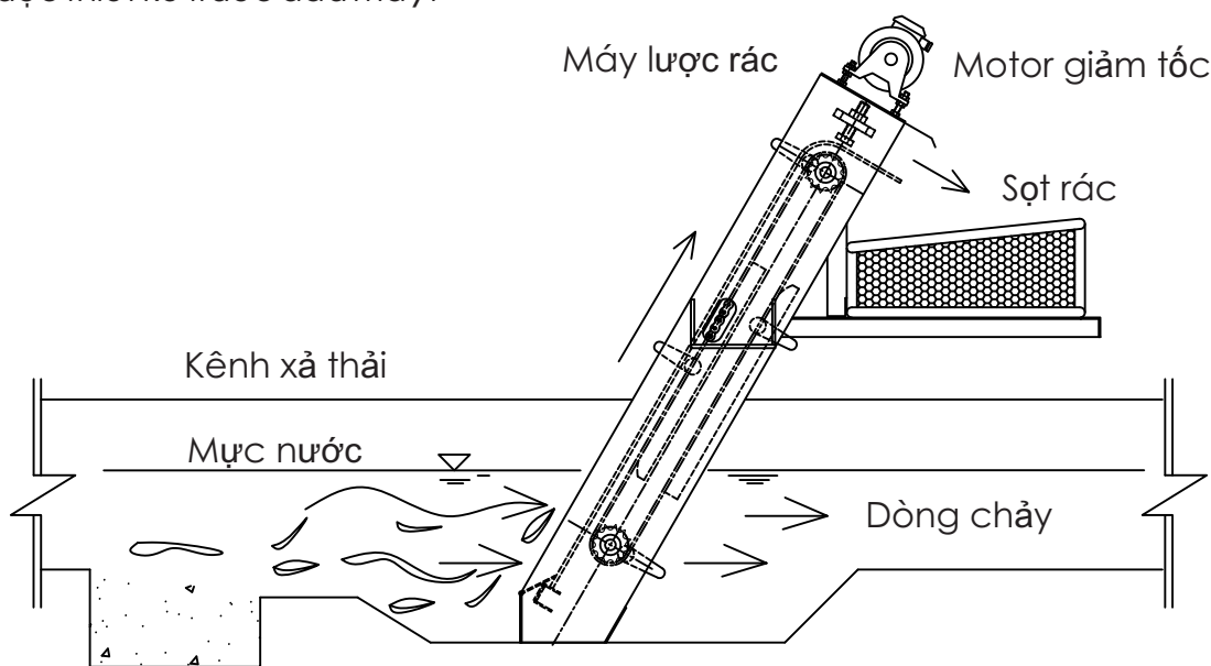
SƠ ĐỒ NGUYÊN LÝ MÁY LƯỘC RÁC
